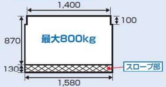
垂直ゲート部 寸法 [単位:mm]
