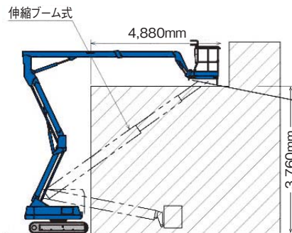
〔NUL工法〕
