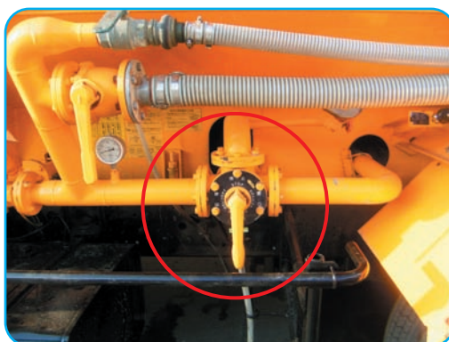
自車汲水・外部散水 切替バルブ
