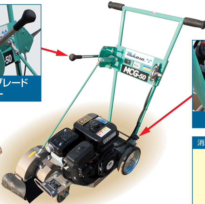
駐車ブレーキ
